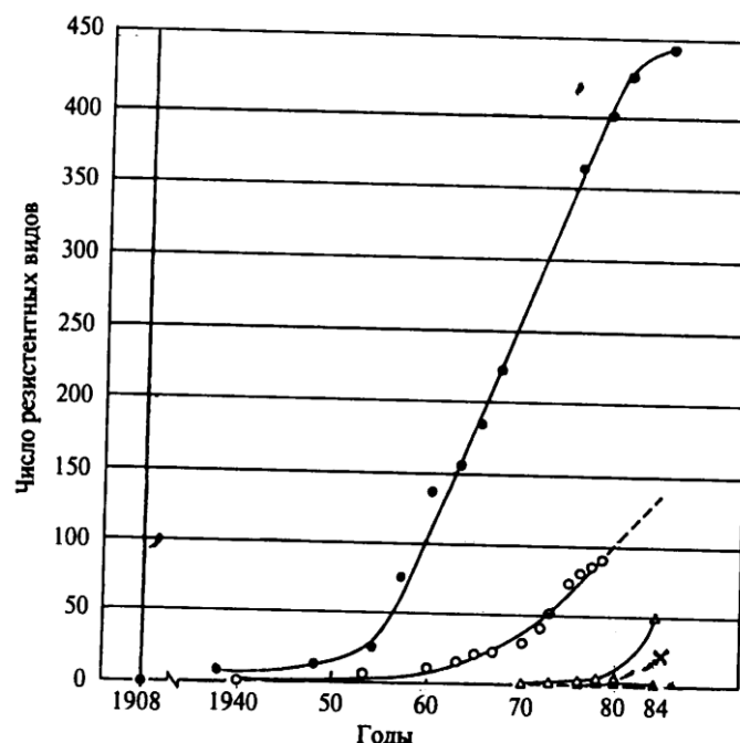
Рис. 1. Динамика развития резистентности к пестицидам у вредных организмов в 1950....84 (Fernandes-Cornejo, Knok, 1998). • -членистоногие, ° - возбудители болезней, Δ - нематоды, х – грызуны.
